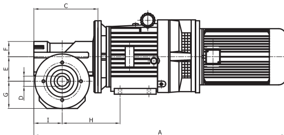
Riduttore P085-P110 Gear-box P085-P110
