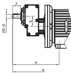
Riduttore 511 Gear-box 511
