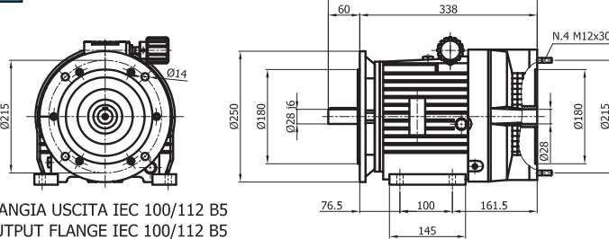
FORMA TYPE 11 ALBERO INGRESSO FEMMINA INPUT FEMALE SHAFT
